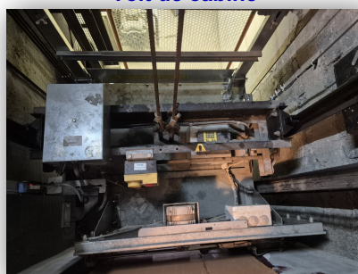
Toit de cabine
